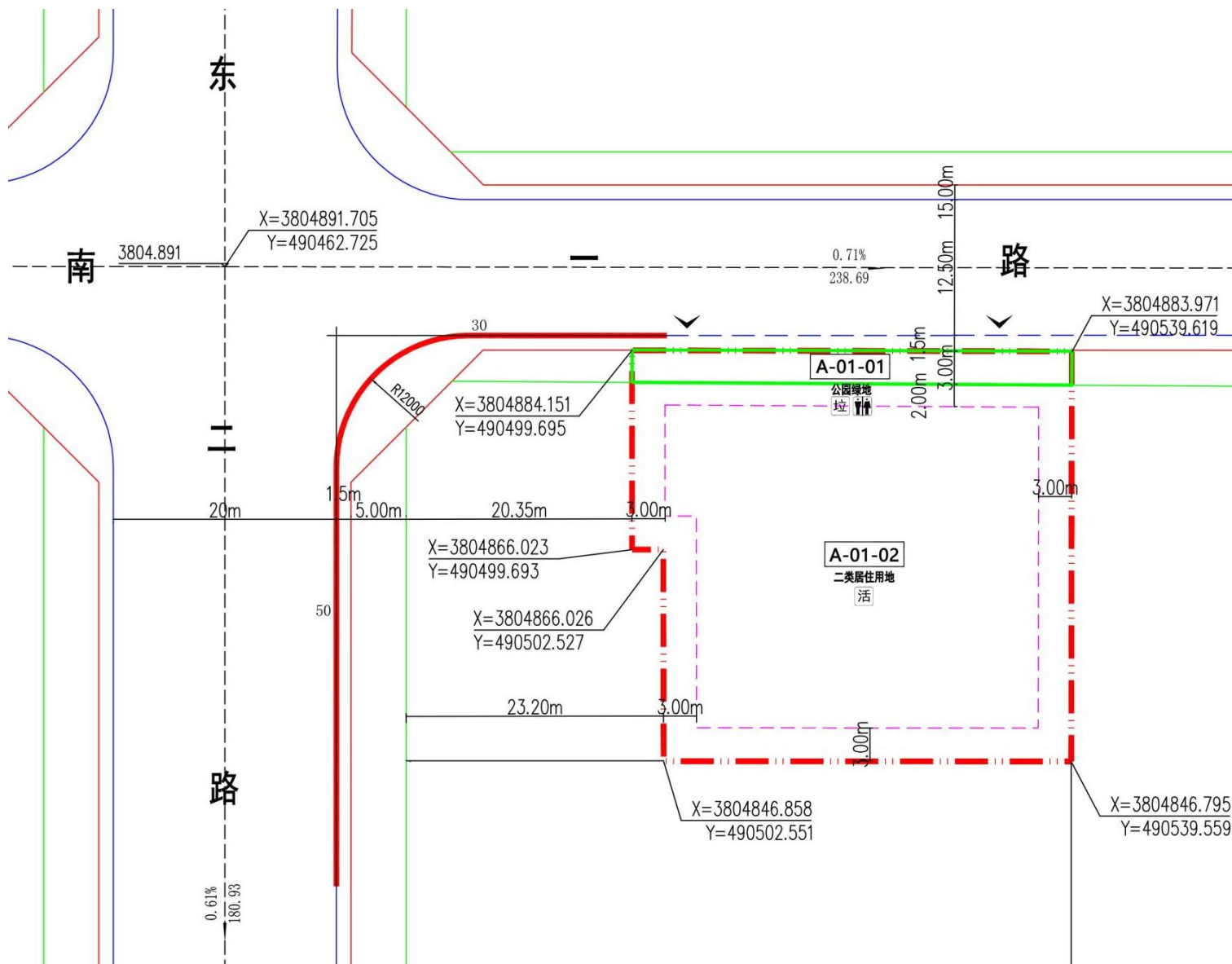
地块位置示意图
