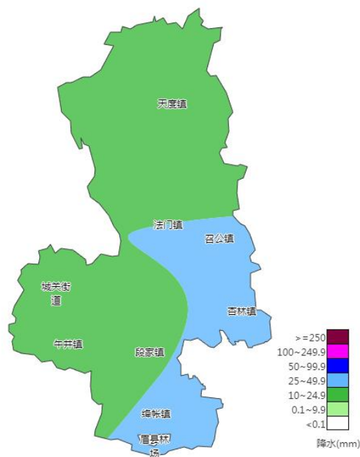
2023-09-18 20:00至2023-09-20 07:00 降水(单位:mm)
